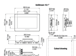
fig. 1. Abmessungen (mm)
