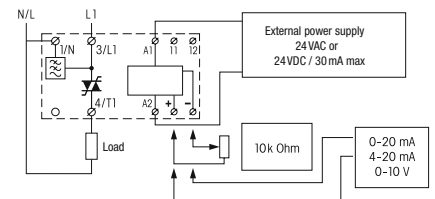
fig. 1. Verdrahtungsdiagramm
