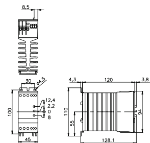
fig. 2. Abmessungen (mm)
