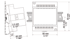
fig. 1. Abmessungen (mm)
