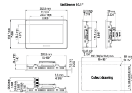
fig. 1. Abmessungen (mm)
