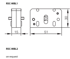
fig. 1. Abmessungen (mm)
